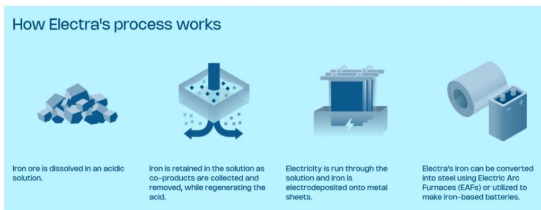
圖 1、Electra 煉鐵過程技術
