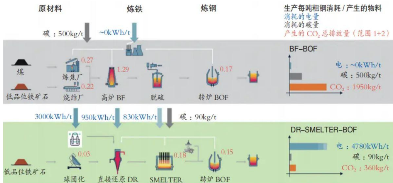
圖 2、傳統高爐-轉爐與 H2DRI-熔爐-轉爐技術路線比較
